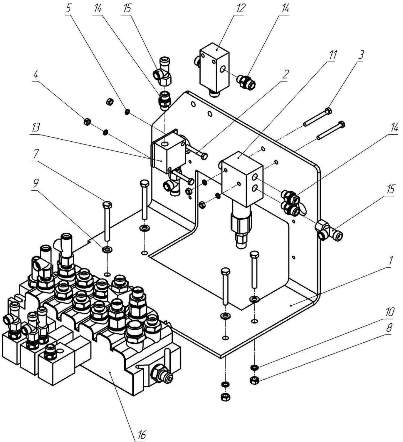
Рисунок 18 – Панель управления
