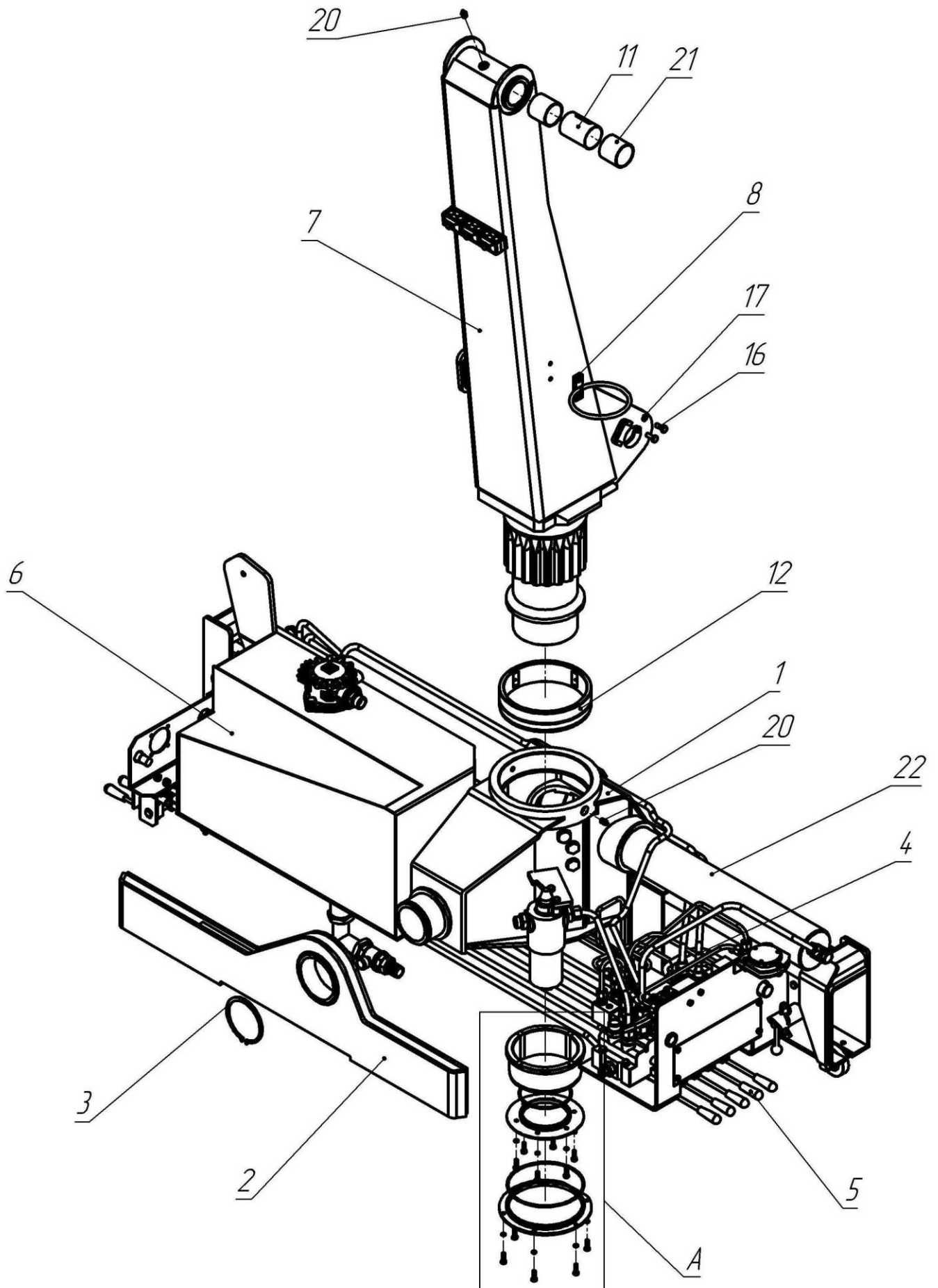
Рисунок 6 – Устройство опорно-поворотное
